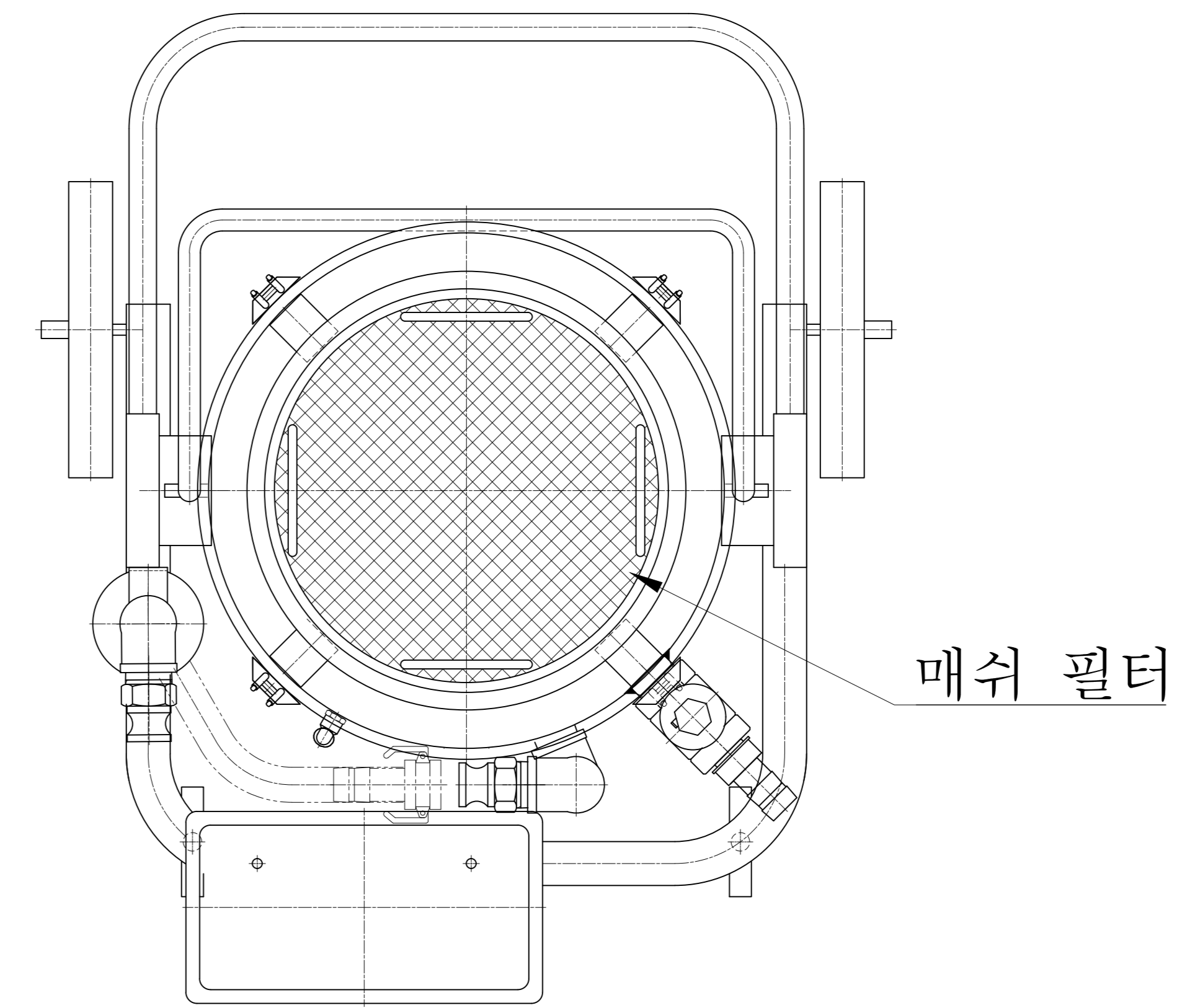
SECTION A-A
